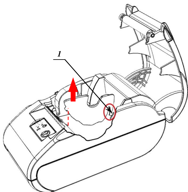
Рисунок 11. Извлечение фиксатора-защелки из паза в лотке ЧЛ
