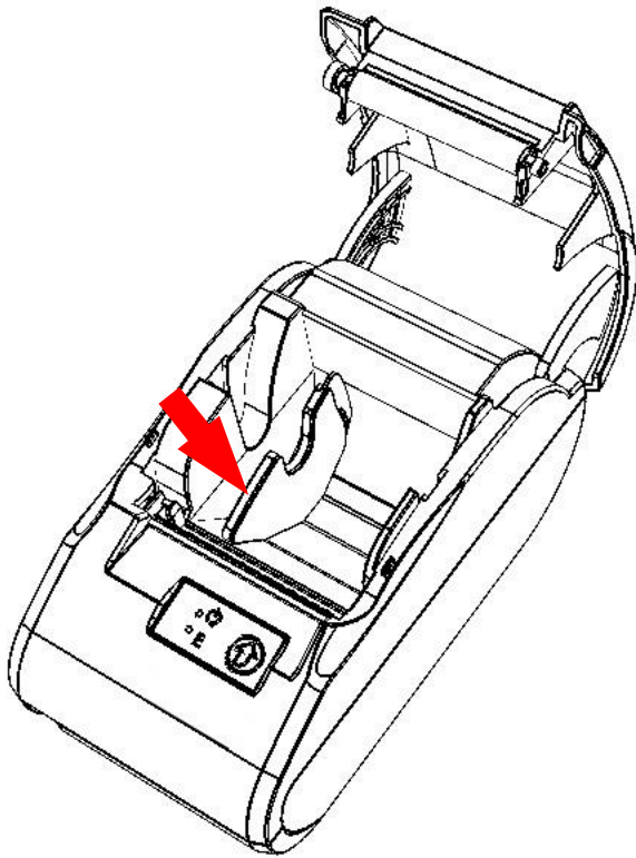
Рисунок 9. Направление приложения усилий при установке ограничителя
