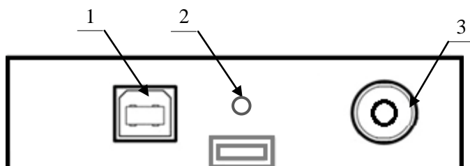
Рисунок 4. Разъемы для подключения внешних устройств к ККТ
